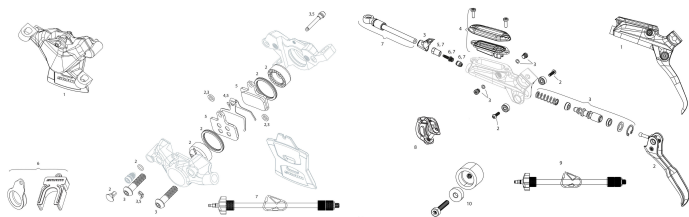
Scheibenbremsen
